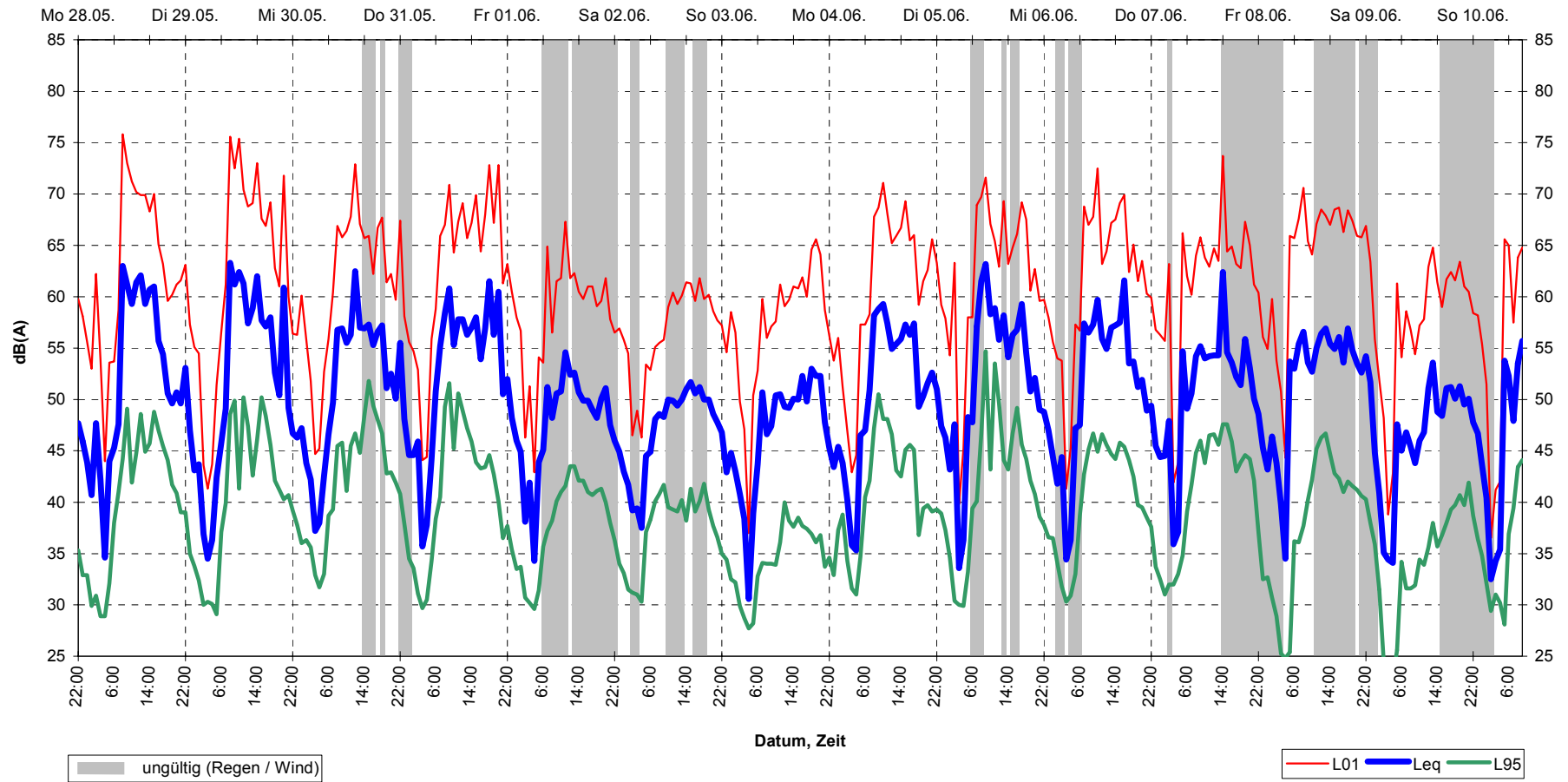
Schalldruckpegel (Stundenmittel) Ostfildern, MP28 28.05.01 bis 11.06.01
