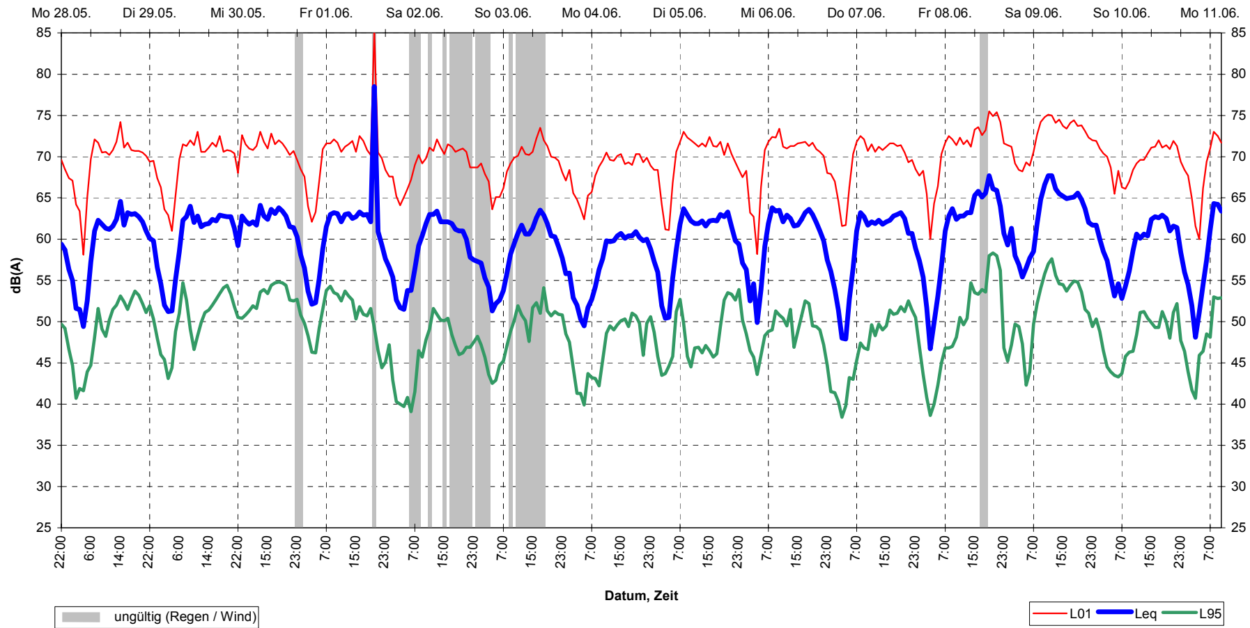
Schalldruckpegel (Stundenmittel) Leinf.-Echterd., MP29 28.05.01 bis 11.06.01
