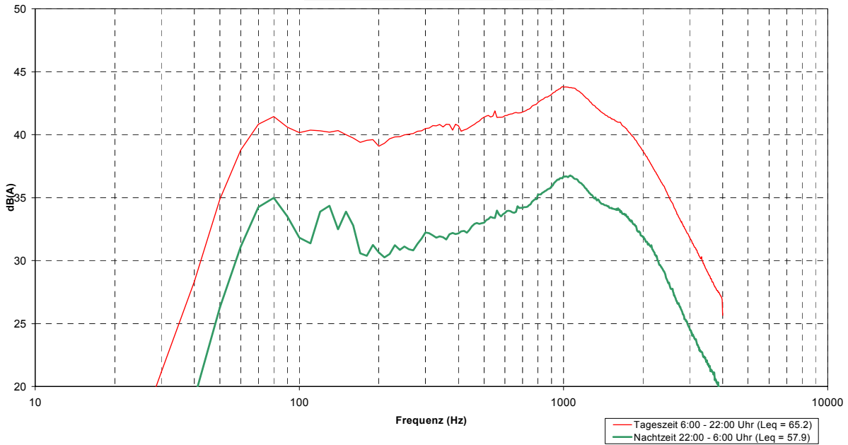
gemittelte Spektren aller gültigen Messungen Leinf.-Echterd., MP31, 21.06.01 bis 25.06.01
