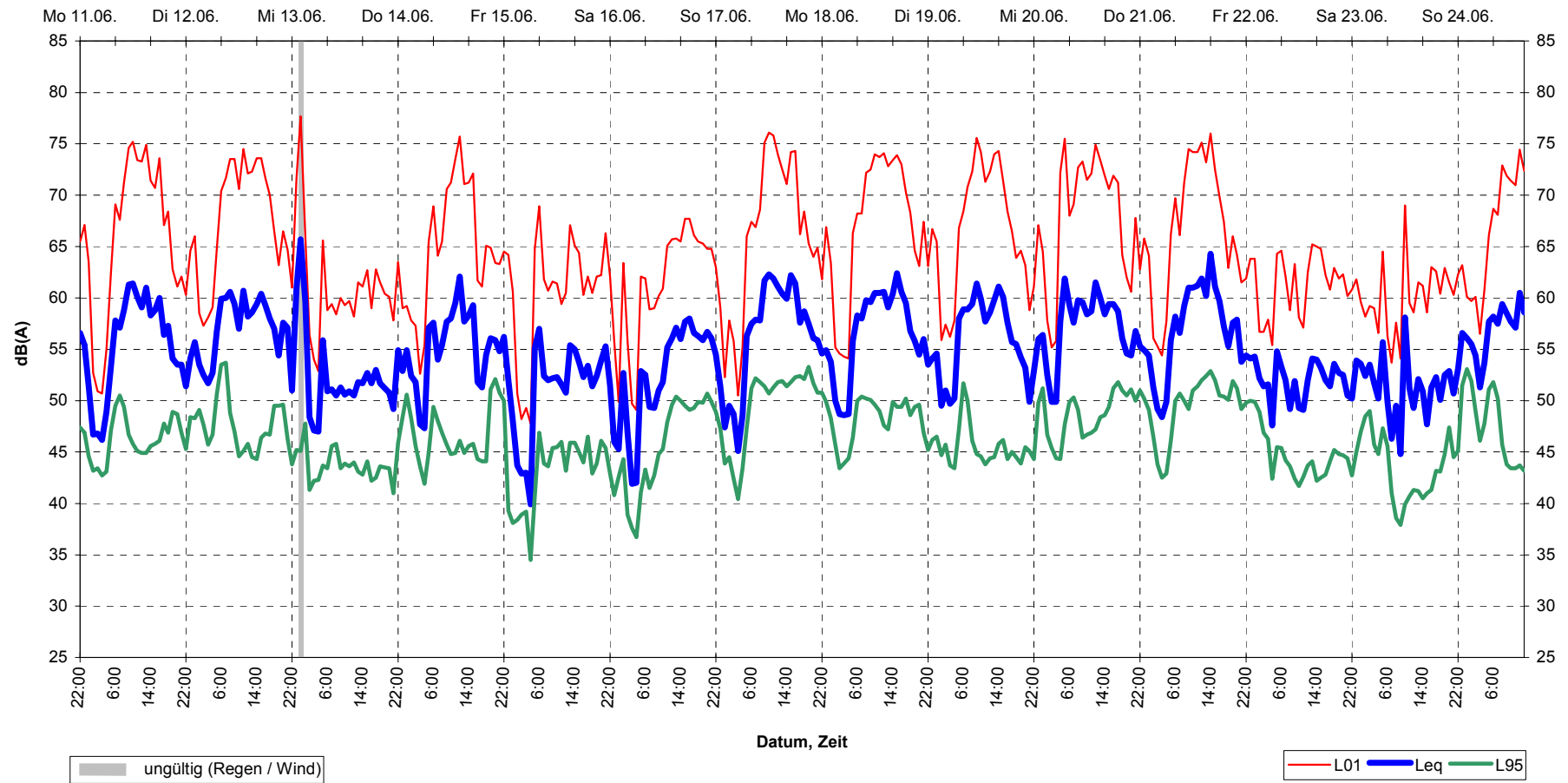
Schalldruckpegel (Stundenmittel) Leinf.-Echterd., MP32 11.06.01 bis 25.06.01
